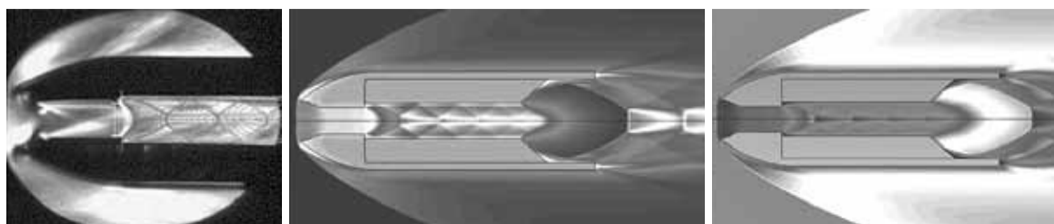
■ Сопоставление результатов эксперимента и численных расчетов для модели ПВРД
